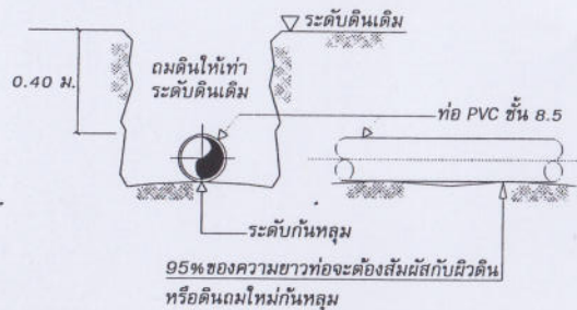
แบบการวางท่อ
